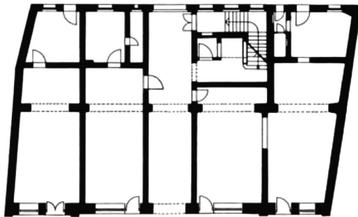
Сл. 2. Основа приземља
